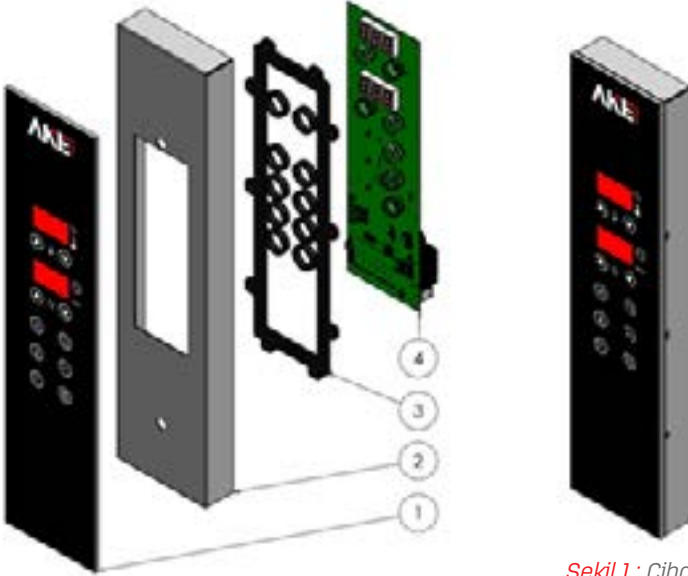
Şekil 1: Cihazın Boyutu ve Montajı
