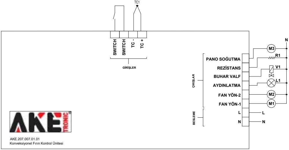
Şekil 2: Elektrik Bağlantı Şeması
